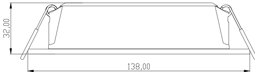
6 寸 15W
